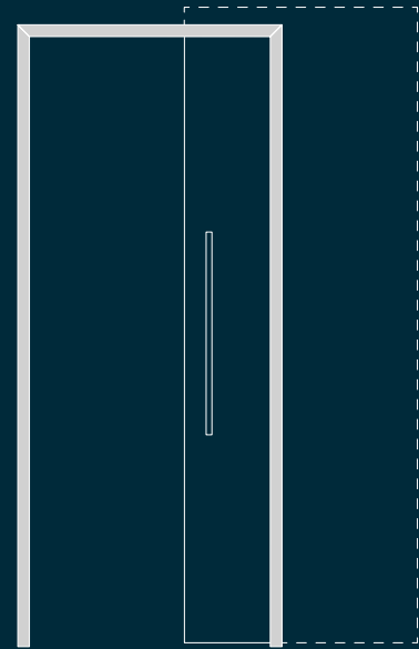
Zarge für In-Wand laufende Schiebetür
